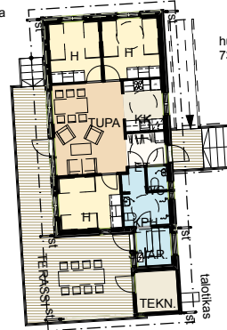
huoneistoala 73,0 m 2
